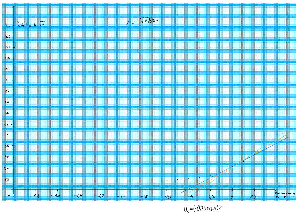
Abbildung 4.5: Ermittlung Sperrspannung für die Spektrallinie bei \lambda = 578 \text{ nm}
